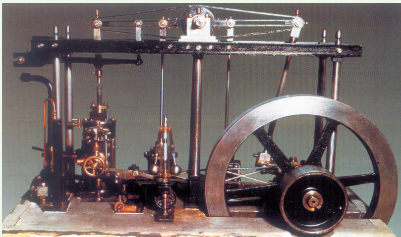
Prima mașină universală industrială cu aburi a lui James Watt construită în 1784
